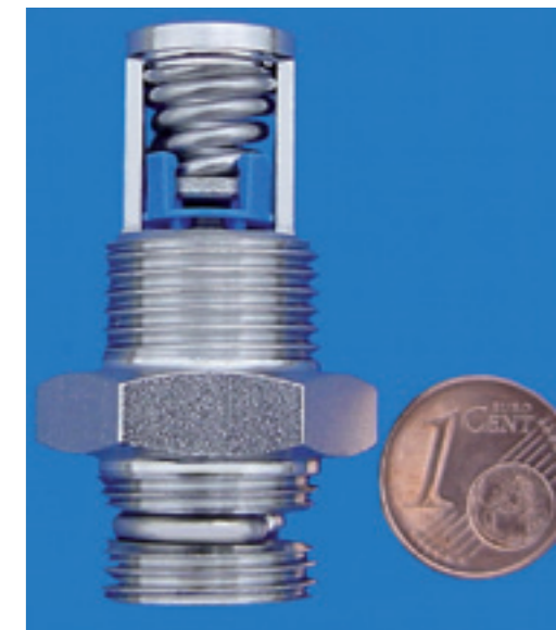
Klein, aber wirksam: Die Elektrolysezelle spaltet Wasser in Wasserstoff, Sauerstoff und Ozon. Das Ozon dient der Wasseraufbereitung
